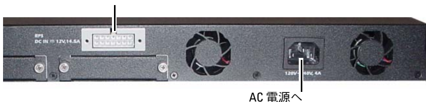
図 1-15. スイッチとの AC/DC 電源接続
